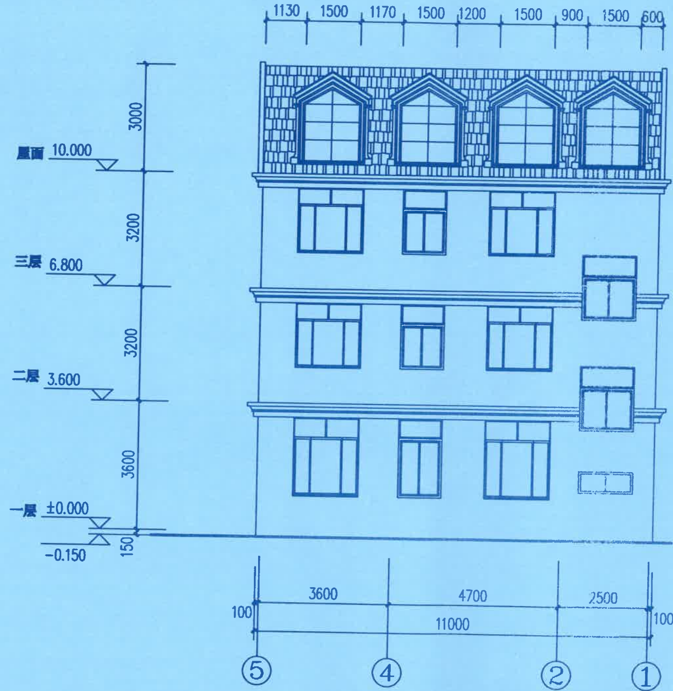
⑤ - ① 轴立面图 1:100
