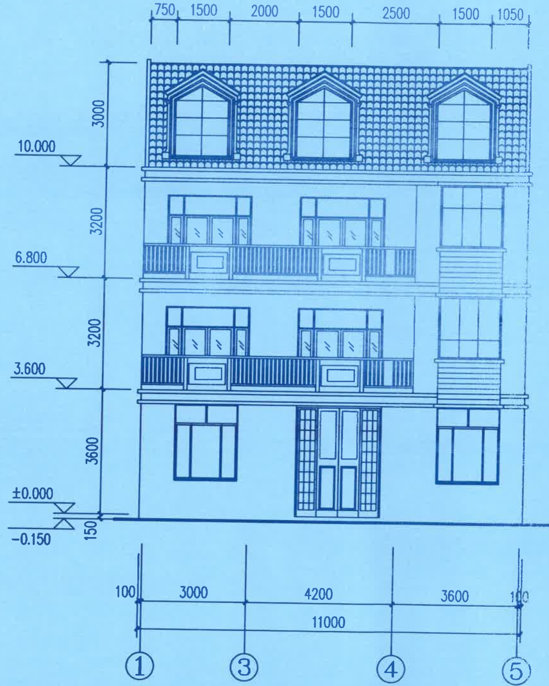
①-⑤轴立面图 1:100
